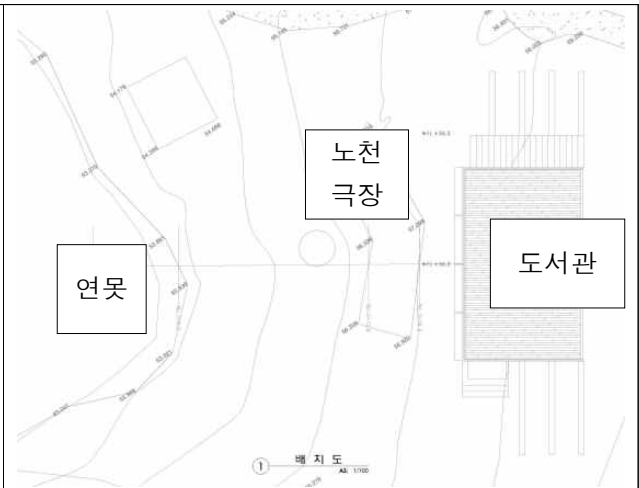
배치도
