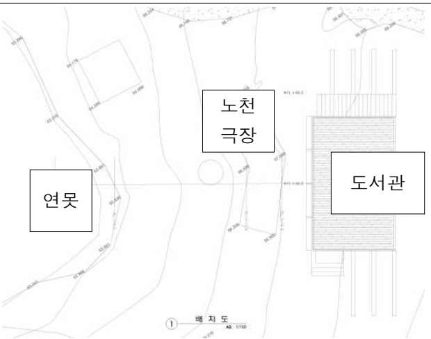
배치도
